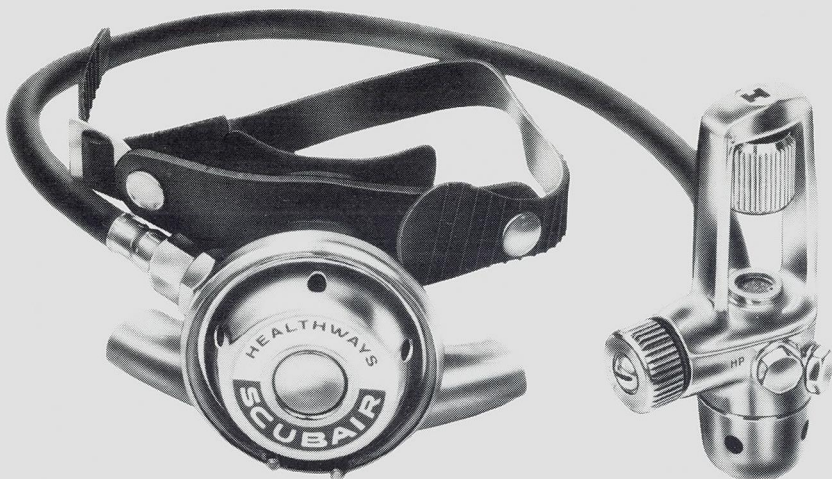
SCUBAIR
