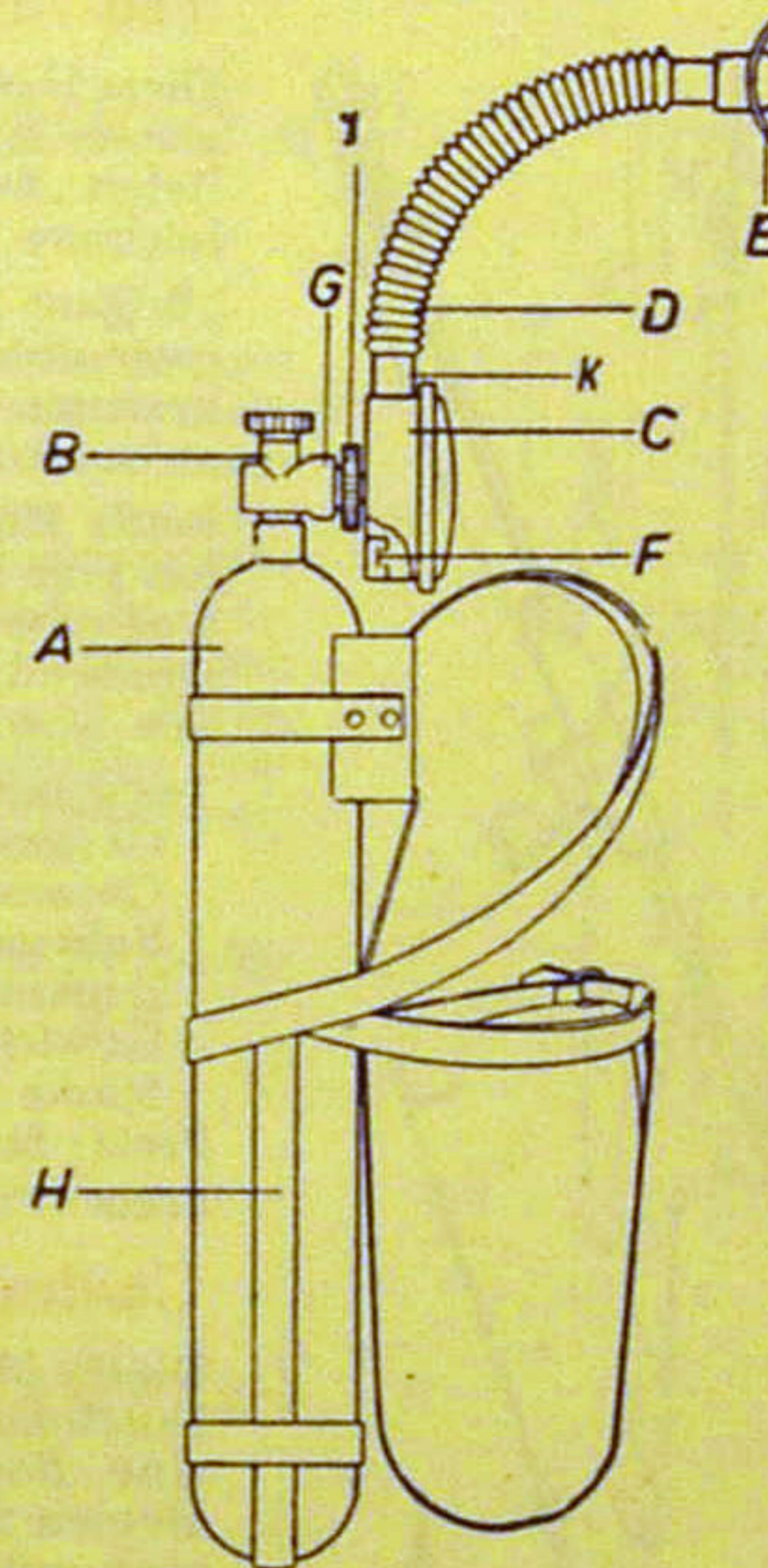
„Delphin II“ Konstruktionszeichnung des 4 Ltr.-Gerätes.
